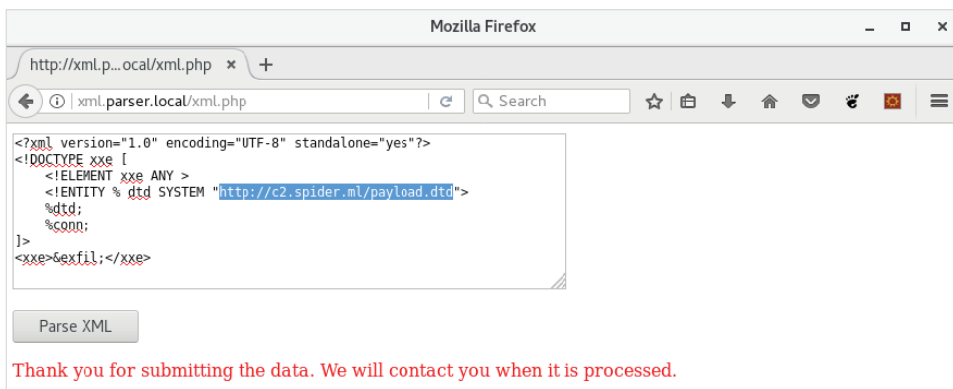
Рис. 10.18. Код модифицированного XML-эксплоита
