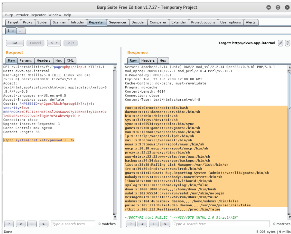
Рис. 5.10. Выполнение кода PHP с использованием локального внедрения файла
