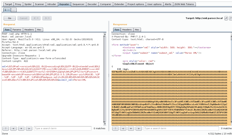
Рис. 10.14. Повторение атаки с использованием модификации PHP-фильтра в кодировке Base64
