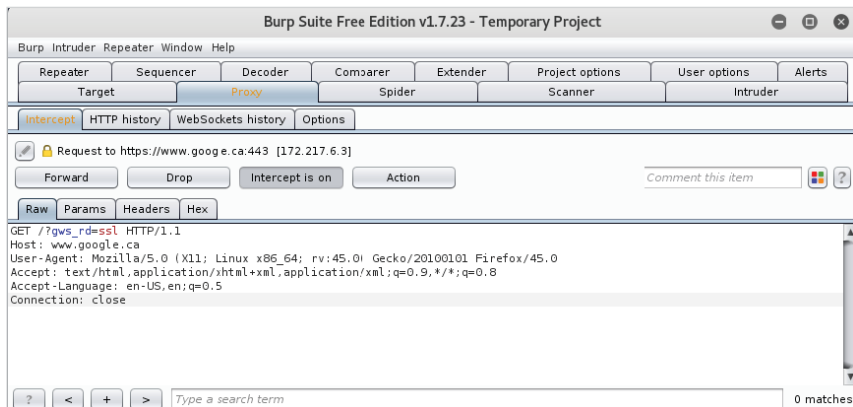
Рис. 1.5. Основной экран бесплатной версии Burp Suite
