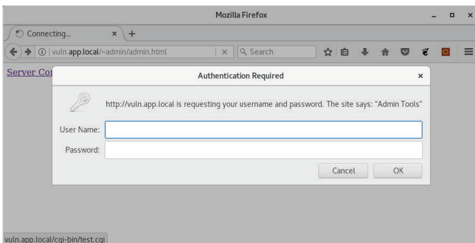
Рис. 2.15. Всплывающее окно аутентификации при попытке перейти по ссылке
