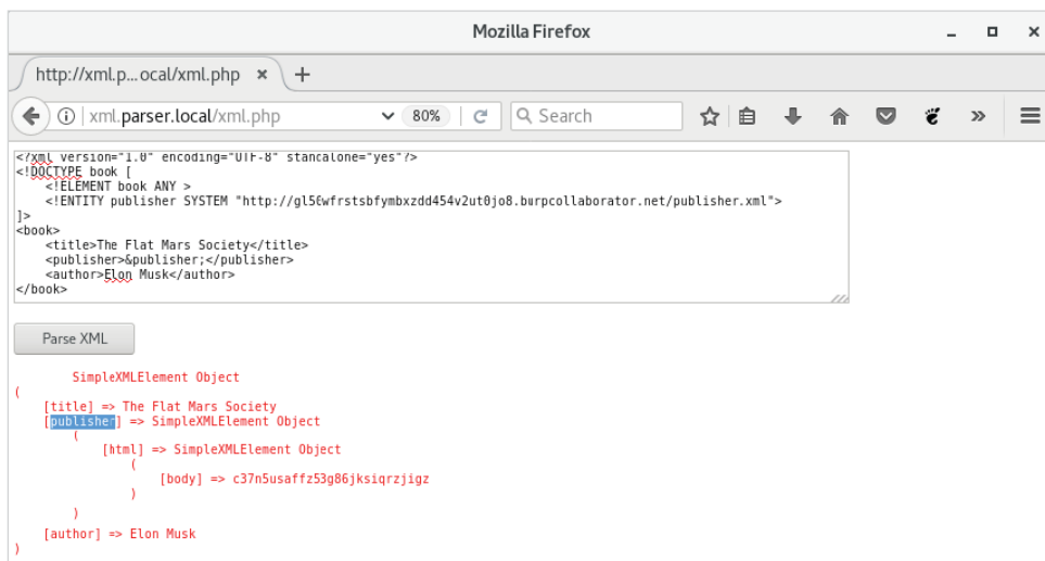
Рис. 10.7. Отправка вредоносного кода XML и наблюдение за ответом
