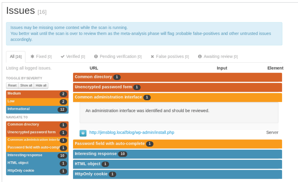
Рис. 12.5. Проблемы, выявленные Arachni
