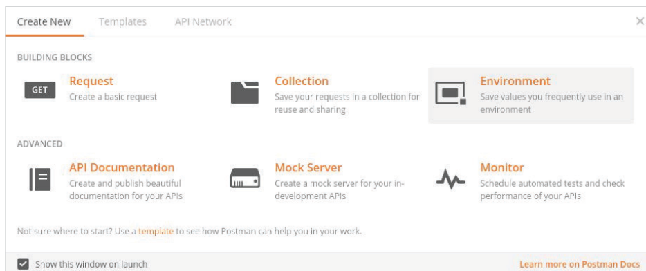
Рис. 11.12. Создание новой среды в Postman
