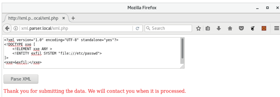
Рис. 10.17. «Слепая» XXE-атака не дает полезного результата
