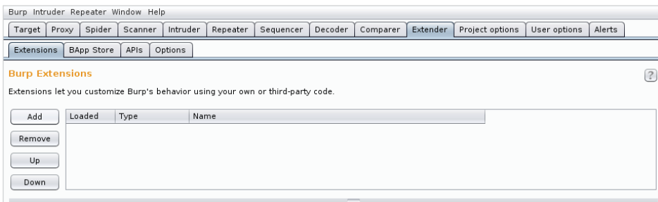
Рис. 11.5. Вкладка Extensions
