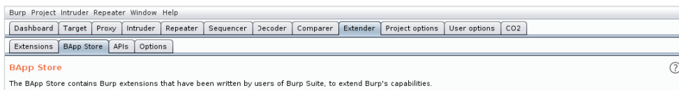
Рис. 7.1. BApp Store
