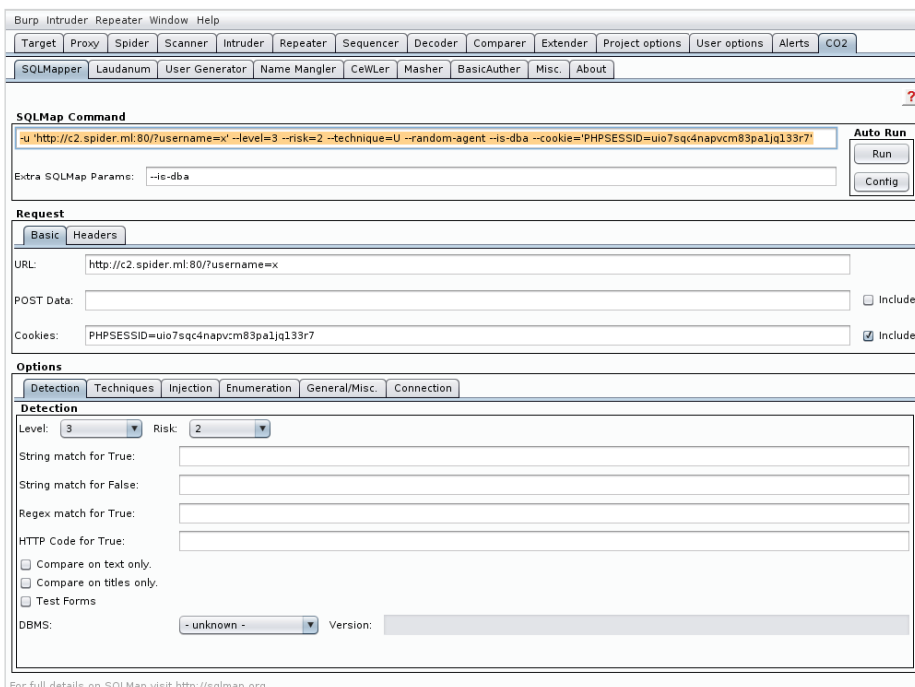
Рис. 7.11. Плагин SQLMapper
