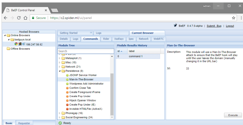
Рис. 9.15. Модуль Man-In-The-Browser
