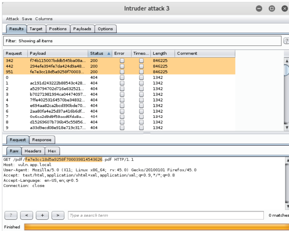
Рис. 2.28. Вкладка Results
