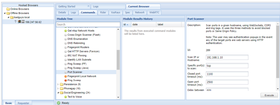
Рис. 9.10. Панель управления сервером ВеЕF
