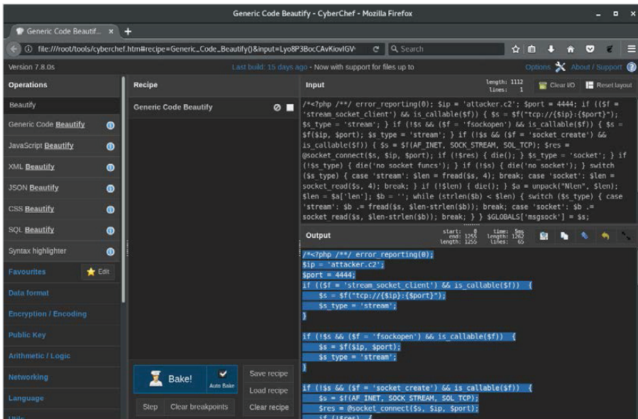
Рис. 12.8. Форматирование кода в CyberChef
