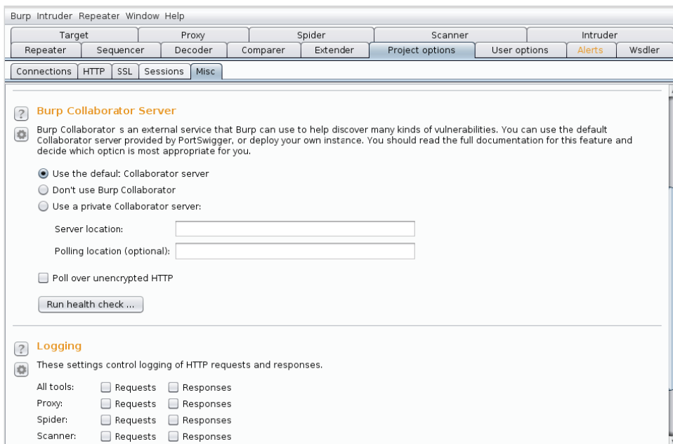
Рис. 7.18. Настройка сервера Collaborator
