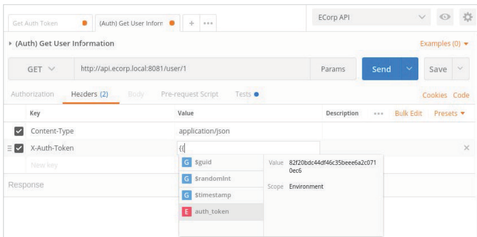
Рис. 11.22. Использование переменных среды в запросах
