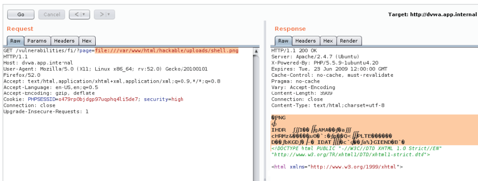
Рис. 5.6. Успешное включение PNG-файла с бэкдором с использованием локального включения файлов
