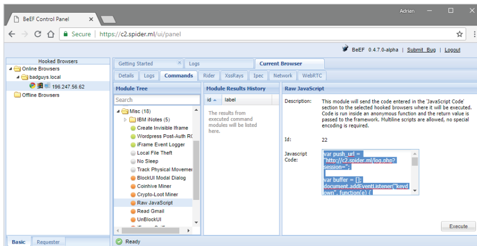
Рис. 9.14. Выполнение пользовательского кейлоггера в перехваченной жертве
