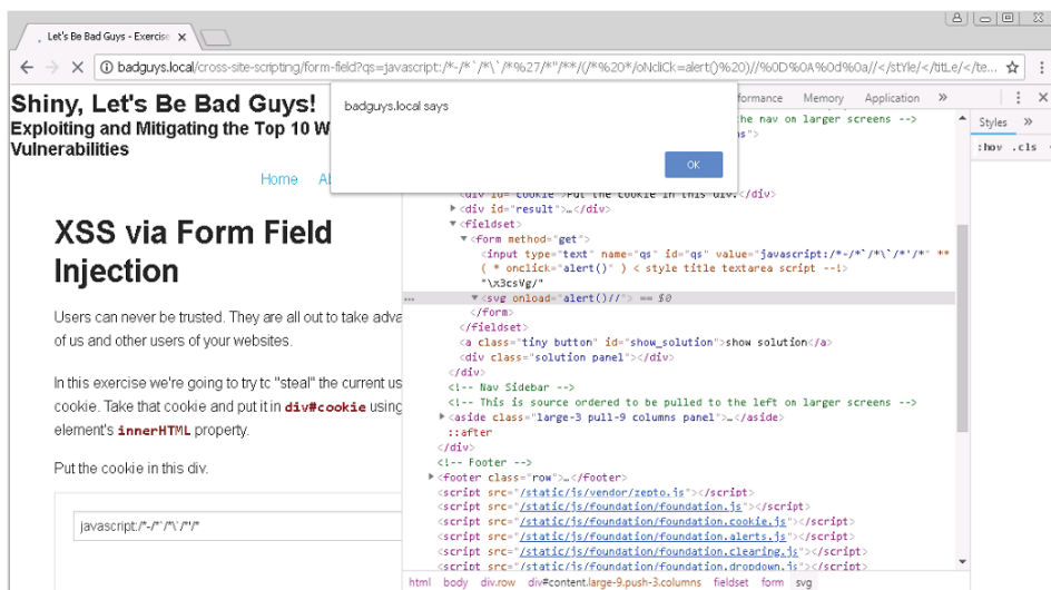
Рис. 9.3. «Полиглот» обнаруживает уязвимость XSS
