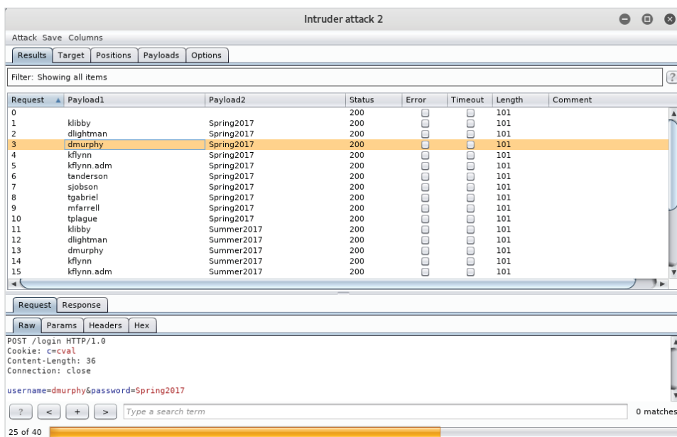
Рис. 4.8. Распыление пароля
