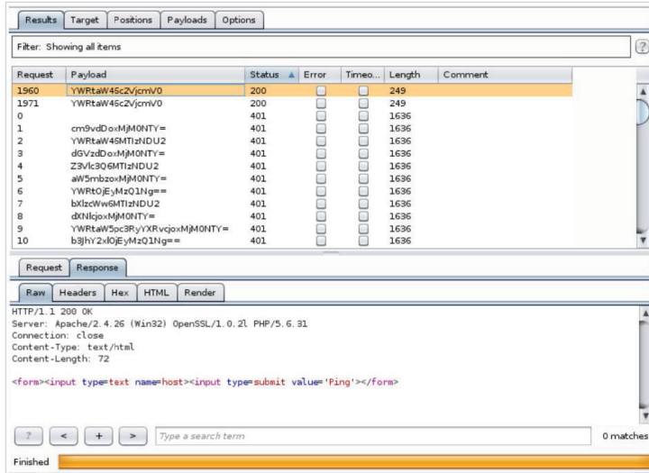
Рис. 2.24. Результаты атаки
