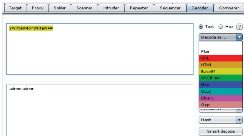
Рис. 2.19. Модуль Decoder
