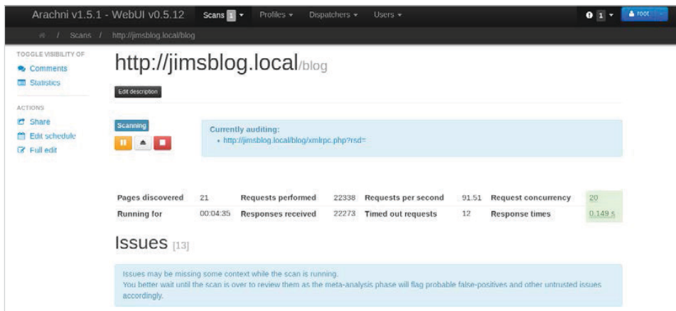
Рис. 12.4. Идет сканирование
