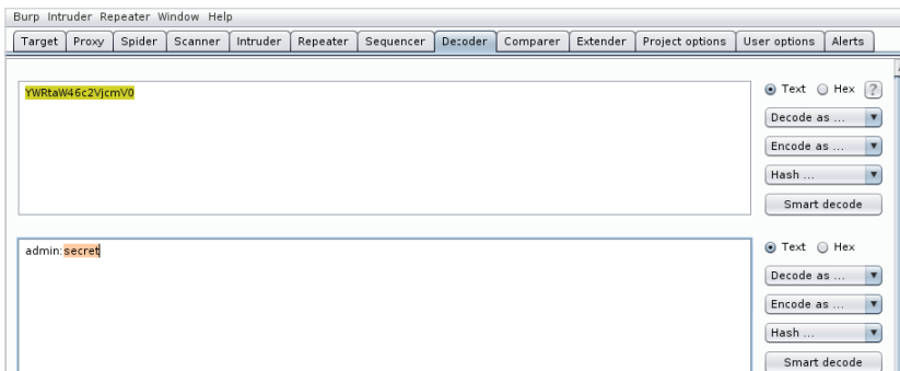
Рис. 2.25. Модуль Decoder
