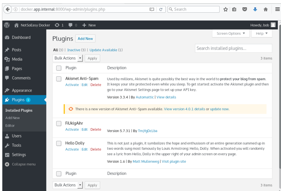
Рис. 13.6. Плагины WordPress
