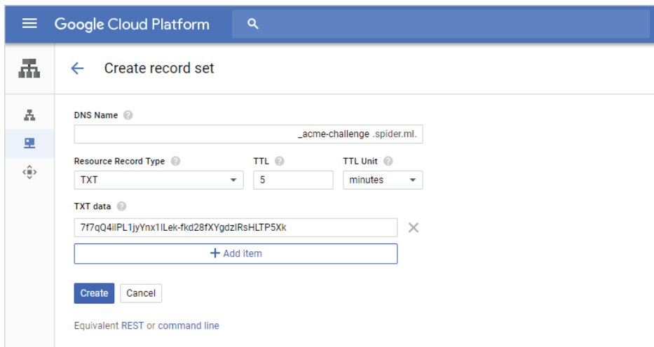
Рис. 6.3. Добавление TXT-записи в DNS
