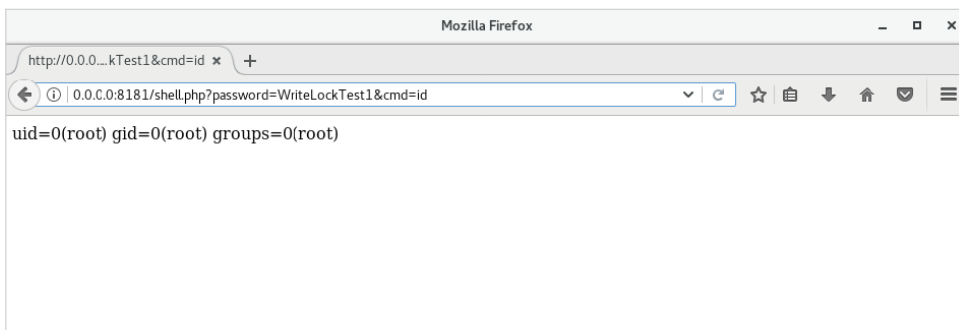
Рис. 8.6. Оболочка успешно выполняет программу id и отображает результат выполнения
