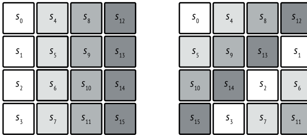
Рис. 4.5. ShiftRows циклически сдвигает байты в каждой строке внутреннего состояния
