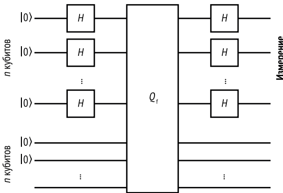
Рис. 14.4. Схема квантового алгоритма, эффективно решающего задачу Саймона
