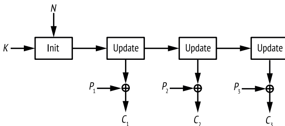
Рис. 5.2. Потоковый шифр с хранимым состоянием
