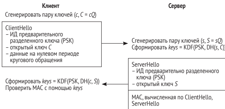
Рис. 13.2. Квитирование при возобновлении сеанса в TLS 1.3. Данные на нулевом периоде кругового обращения посылаются в составе сообщения ClientHello
