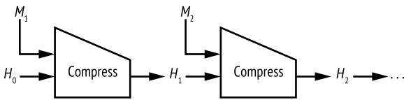
Рис. 6.4. Построение Меркла–Дамгора с использованием функции сжатия Compress
