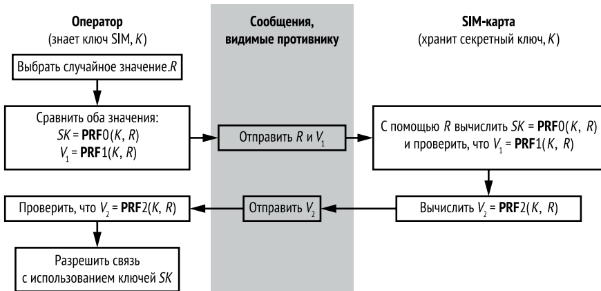
Рис. 11.1. Протокол аутентифицированной выработки ключа в стандартах связи 3G и 4G
