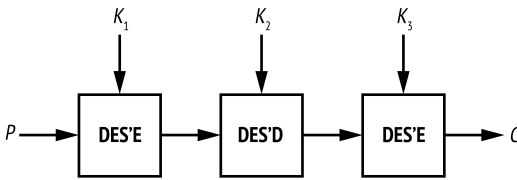
Рис. 4.11. Конструирование блочного шифра 3DES
