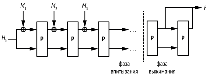
Рис. 6.7. Построение губки
