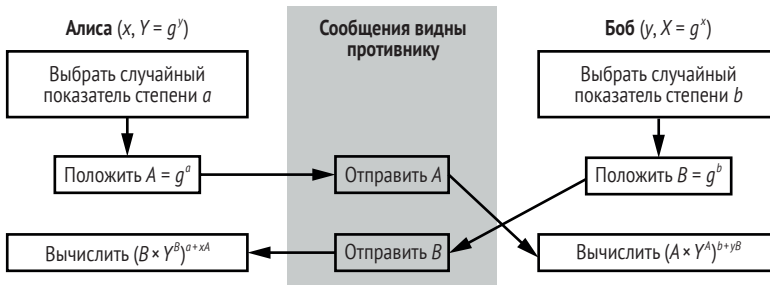
Рис. 11.6. Протокол MQV
