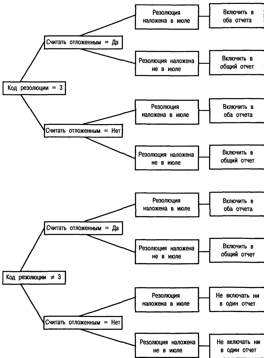
РИСУНОК 12.15. Дерево решений
